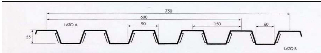
CARICO MASSIMO UNIFORMEMENTE DISTRIBUITO IN Kg/m 2 LG 55/600
